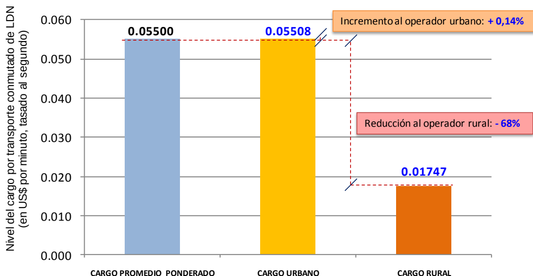
Gráfico N° 7 CARGOS DIFERENCIADOS DE TRANSPORTE CONMUTADO DE LARGA DISTANCIA NACIONAL DE AMÉRICA MÓVIL PERÚ S.A.C.
