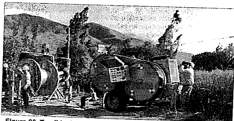
Figura 26. Tendido de cable OPGW con tensión controlada
