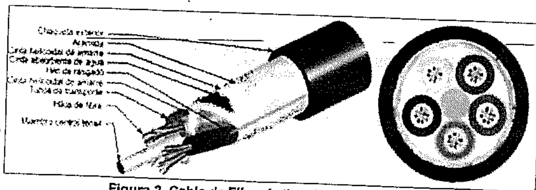
Figura 2. Cable de Fibra óptica tipo ADSS G.652
