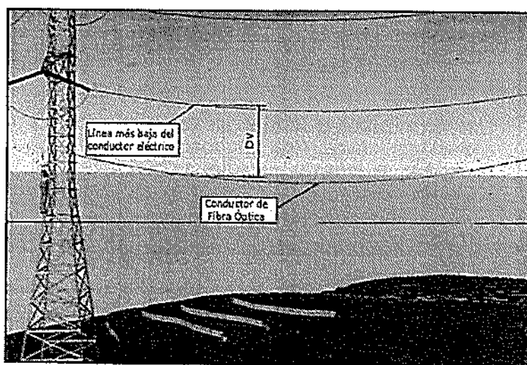
Figura 30. Distancia vertical del cable de FO al conductor
