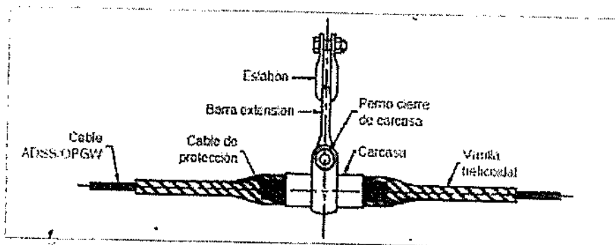
Figura 10. Kit Herraje de Suspensión
