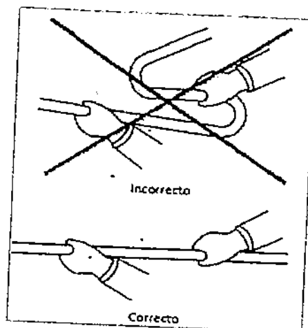
Figura 24. Manera de halar el cable manualmente
