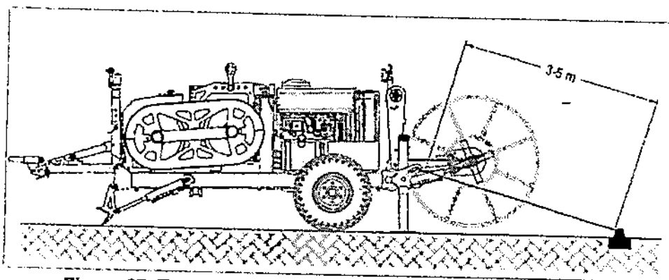
Figura 27. Tendido de cable OPGW con tensión controlada
