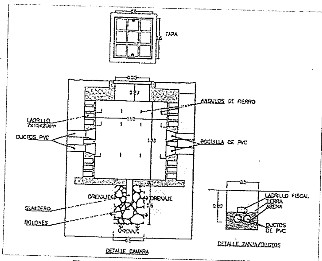
Figura 16. Cámara Existente de electrificadora
