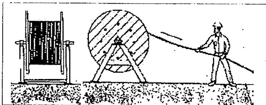
Figura 23. Posición correcta para desenrollar el cable óptico
