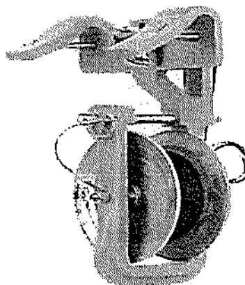
Figura 22. Ejemplo de polea utilizada para tendido aéreo de cable óptico
