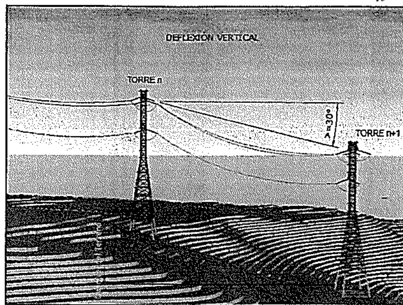
Figura 28. Tendido de cable OPGW con tensión controlada
