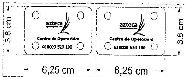
Figura 5. Marquilla externa de Empalme tipo 1
