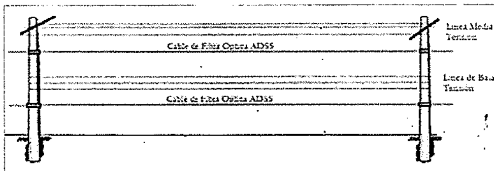
Figura 20. Posición de tendido
