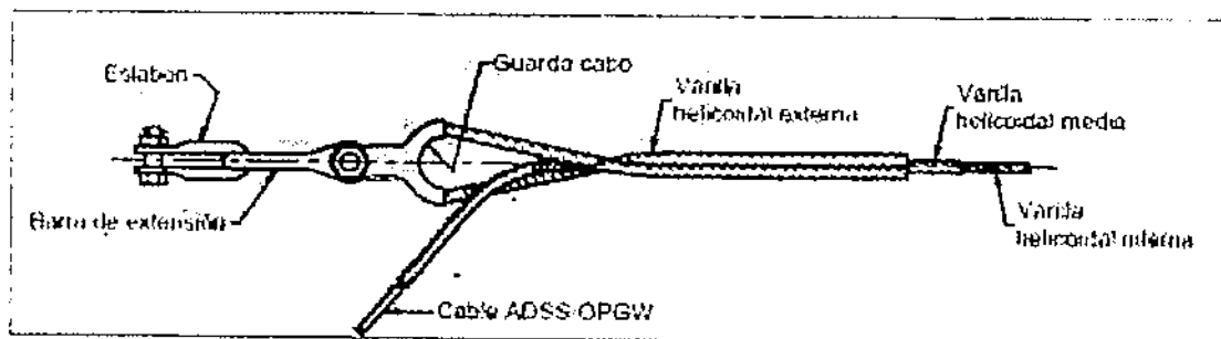
Figura 11. Kit Herraje de Retención
