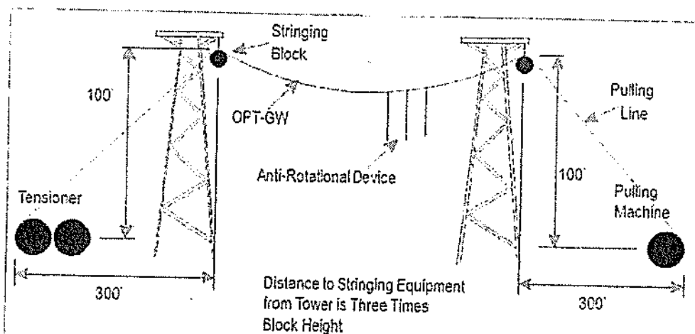
Figura 29. Diagrama ejemplo para Tendido de cable OPGW con tensión controlada
