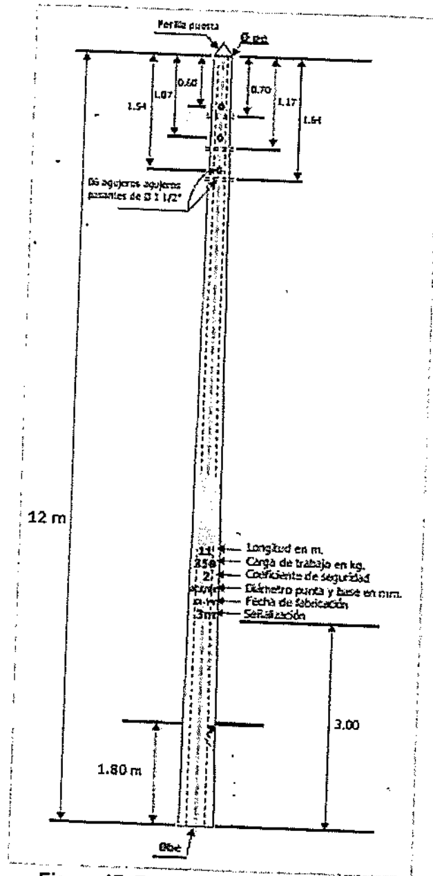
Figura 17. Empotramiento de Posteria
