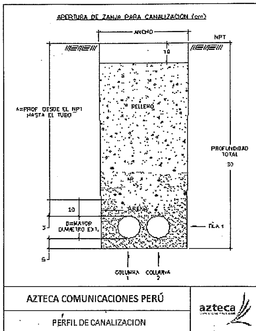
Figura 19. Perfiles de Canalizaciones
