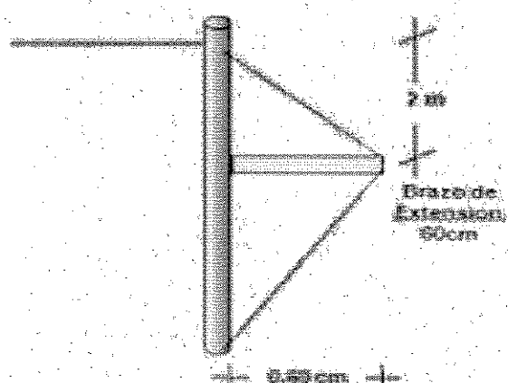
Retenida Especial o Tipo "J"
