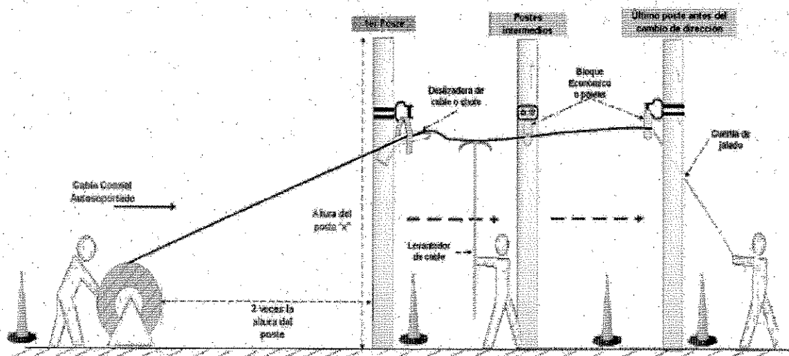
Tendido de Cable
