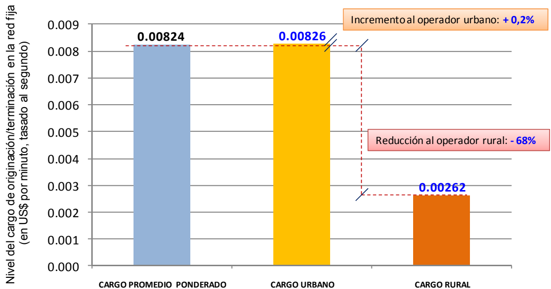
Gráfico N° 3 CARGOS DIFERENCIADOS DE ORIGINACIÓN/TERMINACIÓN EN LA RED DE TELEFONÍA FIJA DE TELMEX PERÚ S.A.
