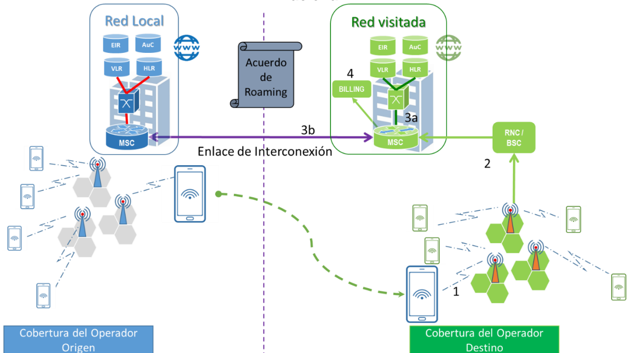
Gráfico N°2: Diagrama de red de un usuario que utiliza el servicio de Roaming Nacional
