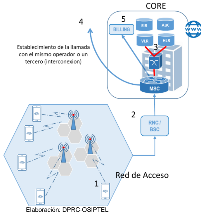
Gráfico N° 1: Diagrama de conexión de un terminal móvil para el establecimiento de una llamada
