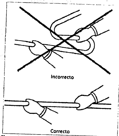
Figura 19. Manera de halar el cable manualmente
