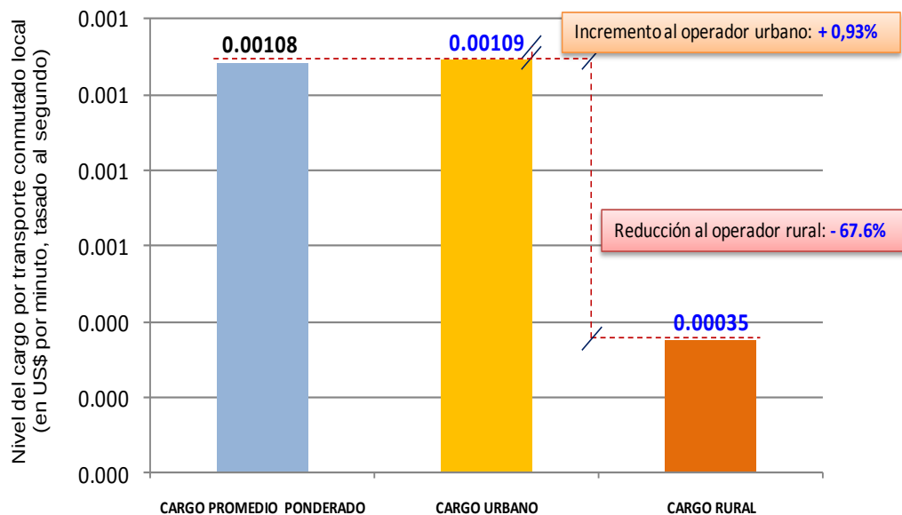
Gráfico N° 6 CARGOS DIFERENCIADOS DE TRANSPORTE CONMUTADO LOCAL DE TELEFÓNICA DEL PERÚ S.A.A.
