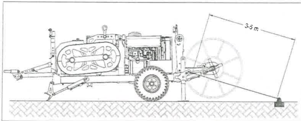
Figura 22. Tendido de cable OPGW con tensión controlada
