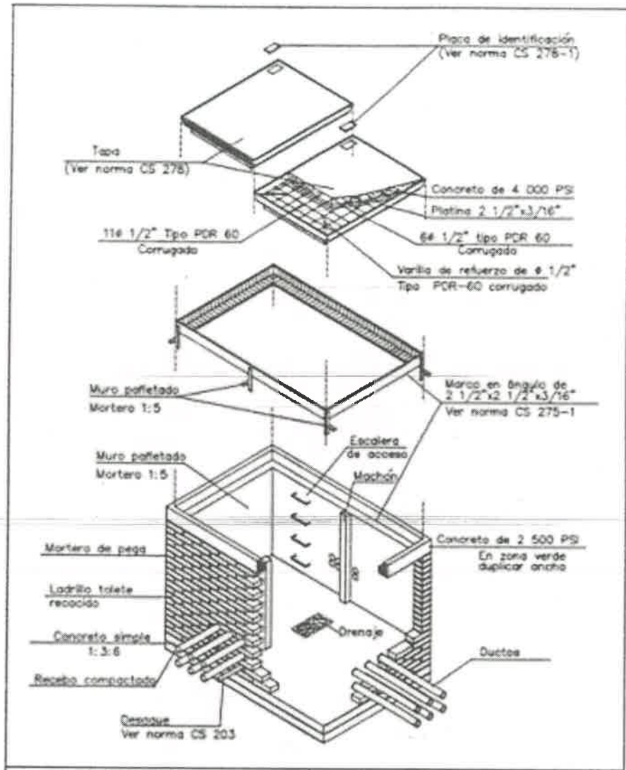
Figura 14. Cámara Existente de electricadora
